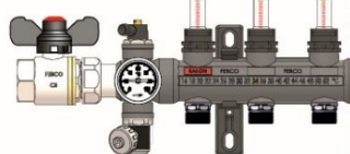
Nuevo modelo con rosca metálica y válvula termostaticable métrica M30
